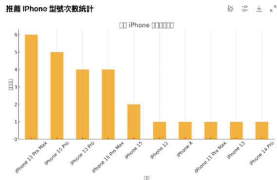
推薦 iPhone 型號次數統計
